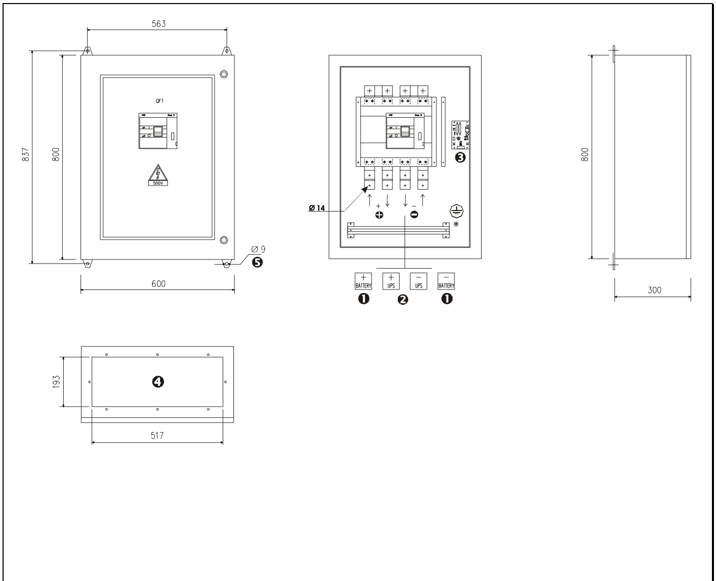
Рисунок 3.10 Блок размыкателя батарей – 630 А
