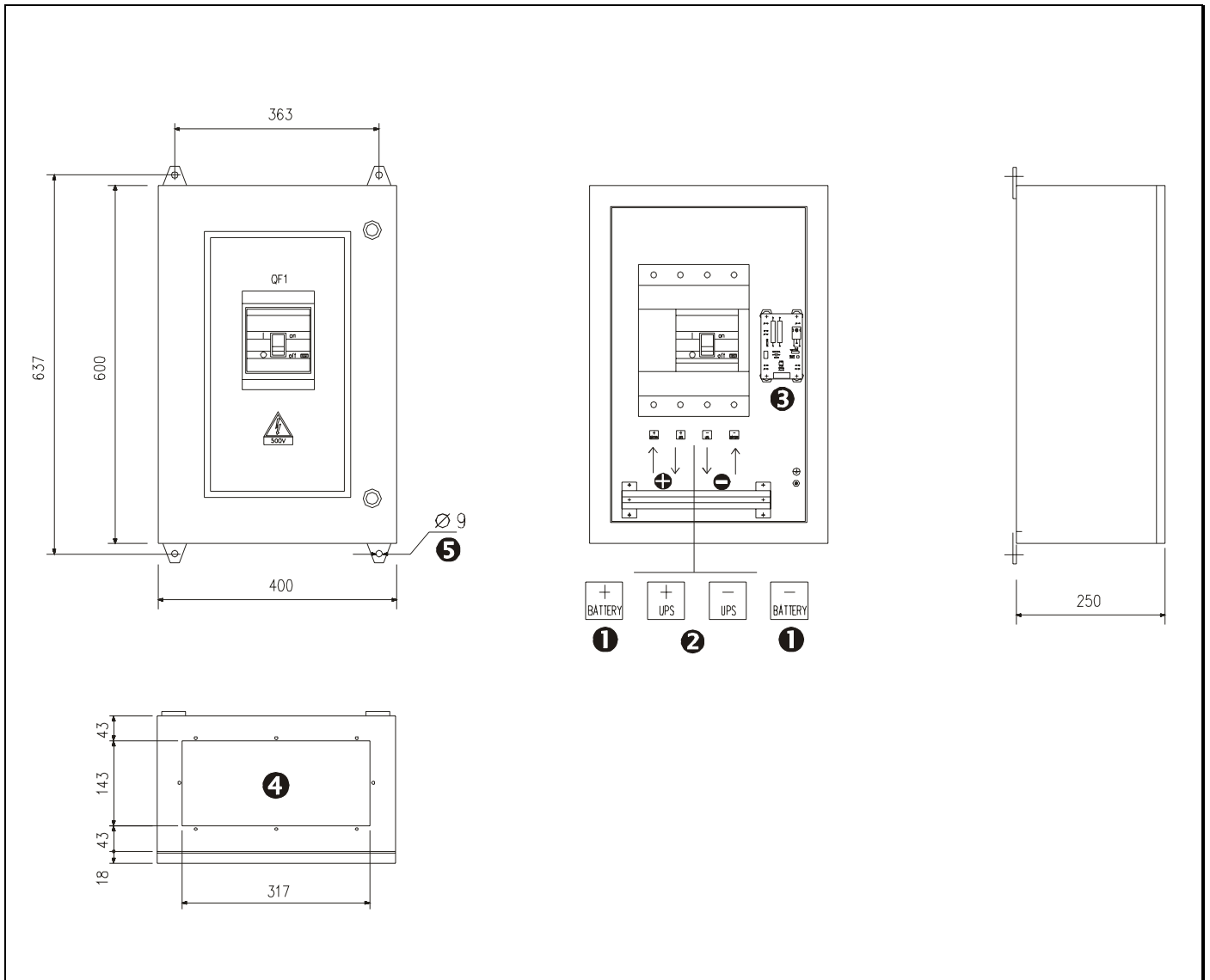
Рисунок 3.9 Блок размыкателя батарей – 400 А
