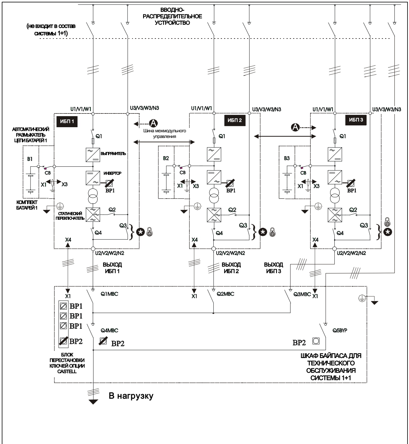
Рисунок 4.9 Пример конфигурации системы из трех ИБП, соединенных параллельно, со шкафом внешнего технического байпаса
