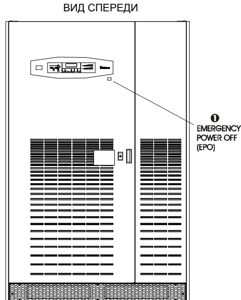
Рисунок 8-3. Кнопка аварийного отключения ИБП (EPO)
