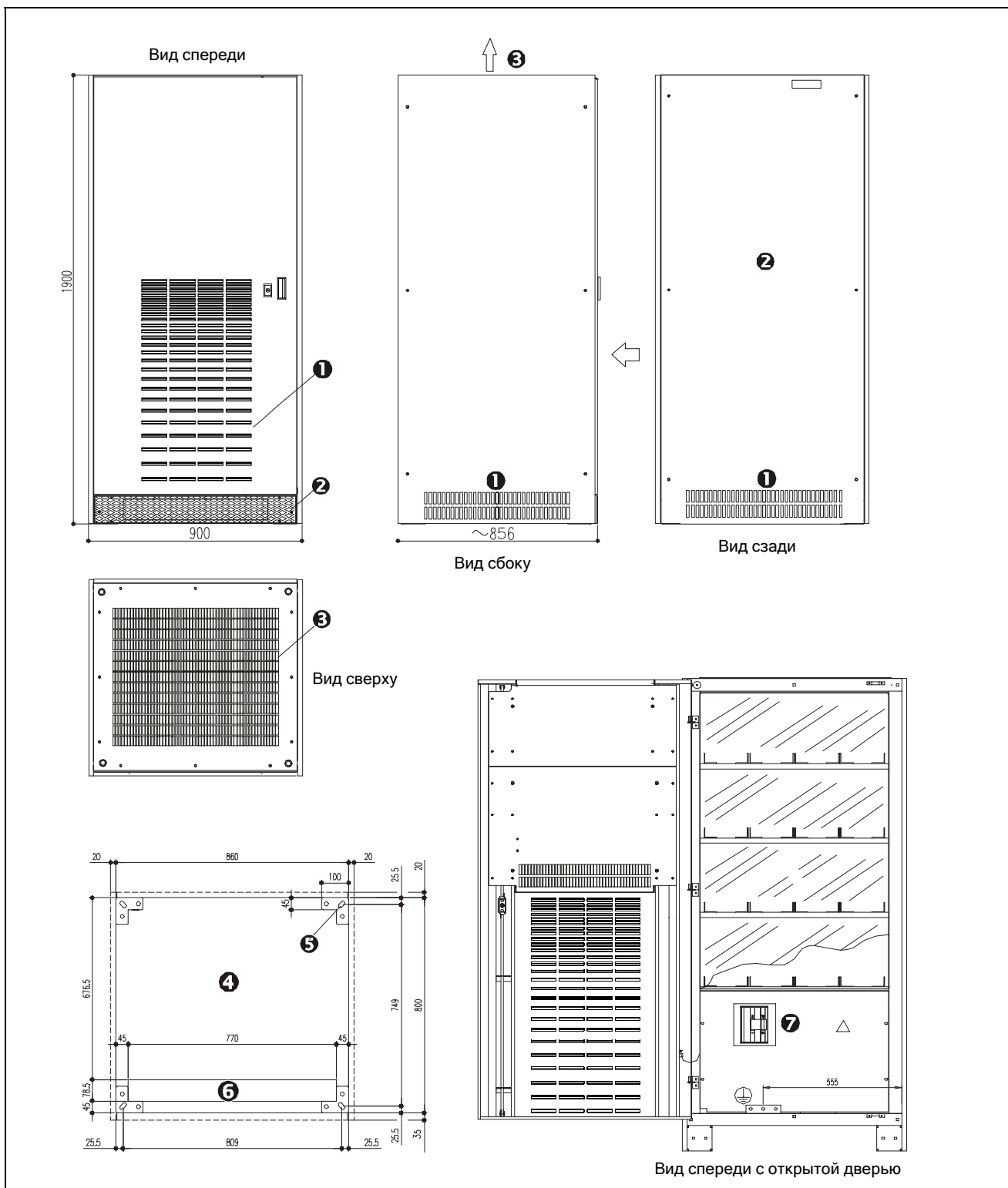
Рисунок 3.6 Батареиный шкаф для ИБП 160/200 кВА
