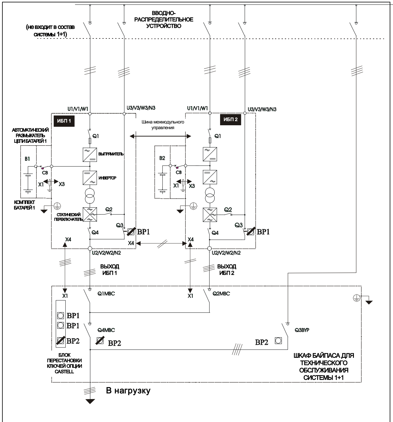
Рисунок 4.8 Схема-пример конфигурации параллельного соединения двух ИБП для избыточности со шкафом внешнего технического байпаса.
