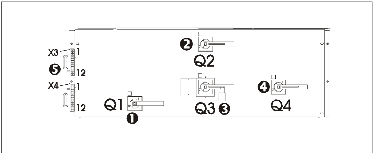
Рисунок 9-1 Расположение силовых выключателей
